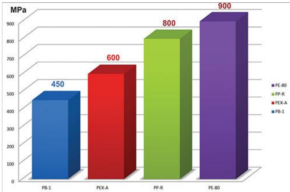
Рисунок 5. Коэффициент эластичности
