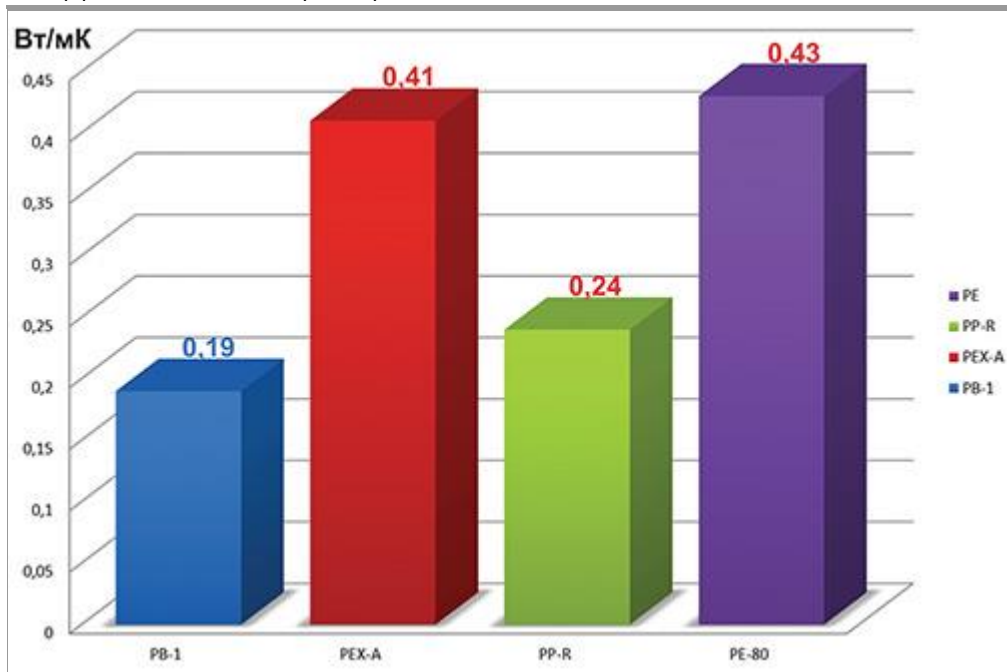
Рисунок 4. Коэффициент теплопроводности
