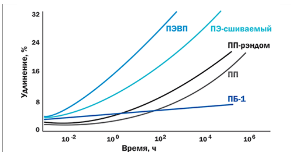
Рисунок 1. Стойкость к деформации под нагрузкой ПБ-1 по сравнению с другими полиолефиновыми материалами
